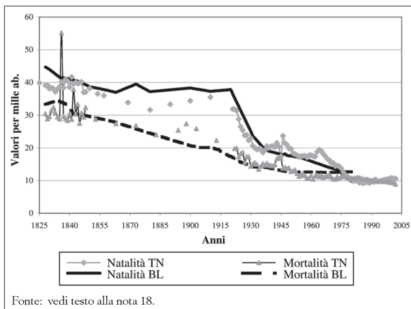
Fig. 3 - Natalità e mortalità in Trentino (1825-2002); confronto con la Provincia di Belluno (1825-1980) (valori per mille ab.).
