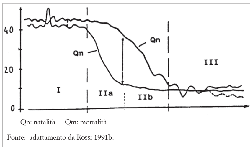
Fig. 2 - Lo schema della transizione demografica.
